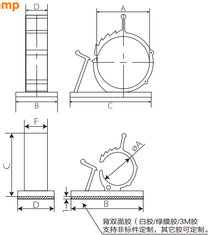
配线固定座 Cable Clamp
