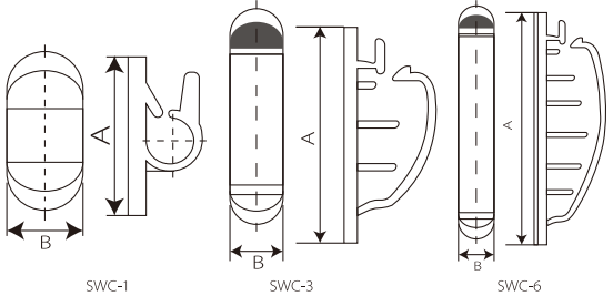
自粘式分位固定座 Cable Clamp
