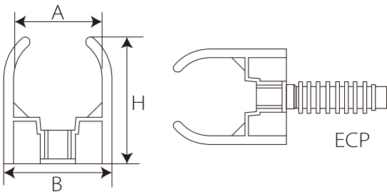
马鞍型管夹 SaddleType Clips
