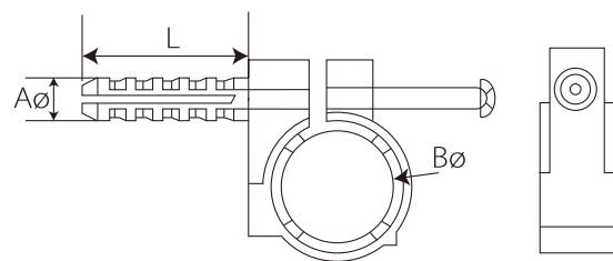
P型膨胀管夹 P Type Clips 材质: PPR。 用途: 用于固定适合外径的管材, 如 PPR管、PVC管, PE管等。 Material: PPR. Usage: Used to fix pipes suitable for outerdiameter, such as PPR pipes,PVC pipes,PE pipes, etc.
